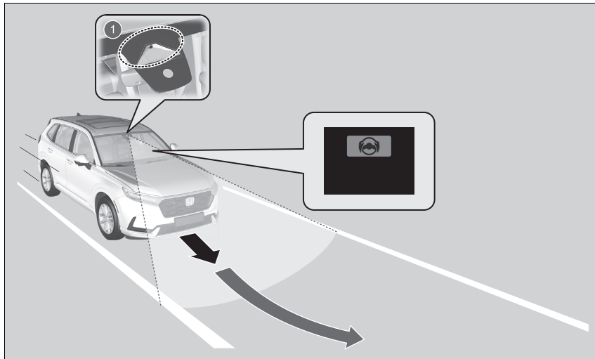
1 Přední snímací kamera: Sleduje podélné čáry jízdního pruhu.
