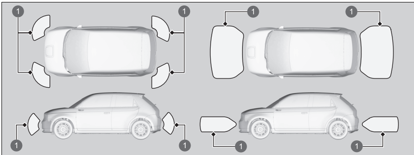
1 Dosah snímače
